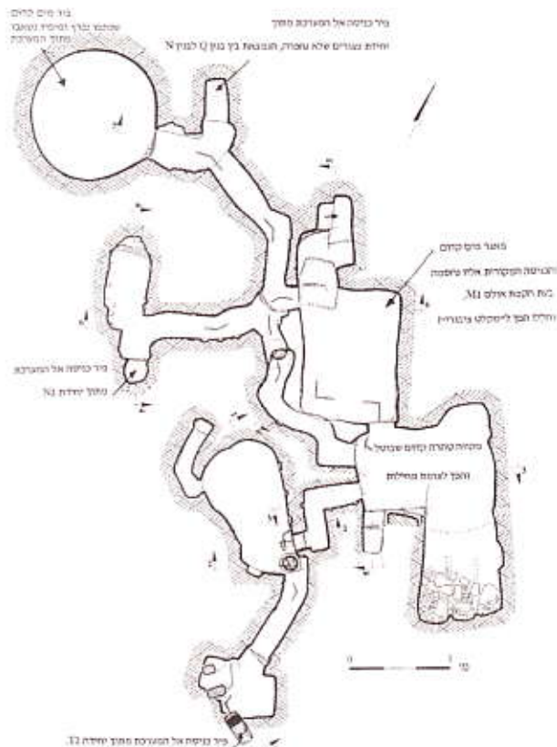
חורבת עתרי; תוכנית מערכת מסתור XV
