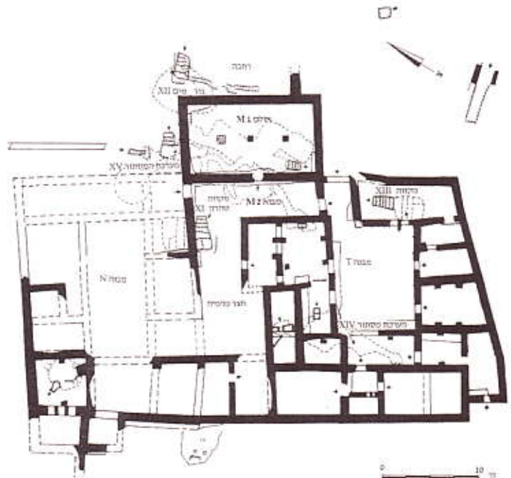
חורבת עתרי; תוכנית מבנה הציבור M ומבני המגורים הסמוכים אליו בתקופה שבין המרידות נגד הרומאים (70-135 לסה"נ)
